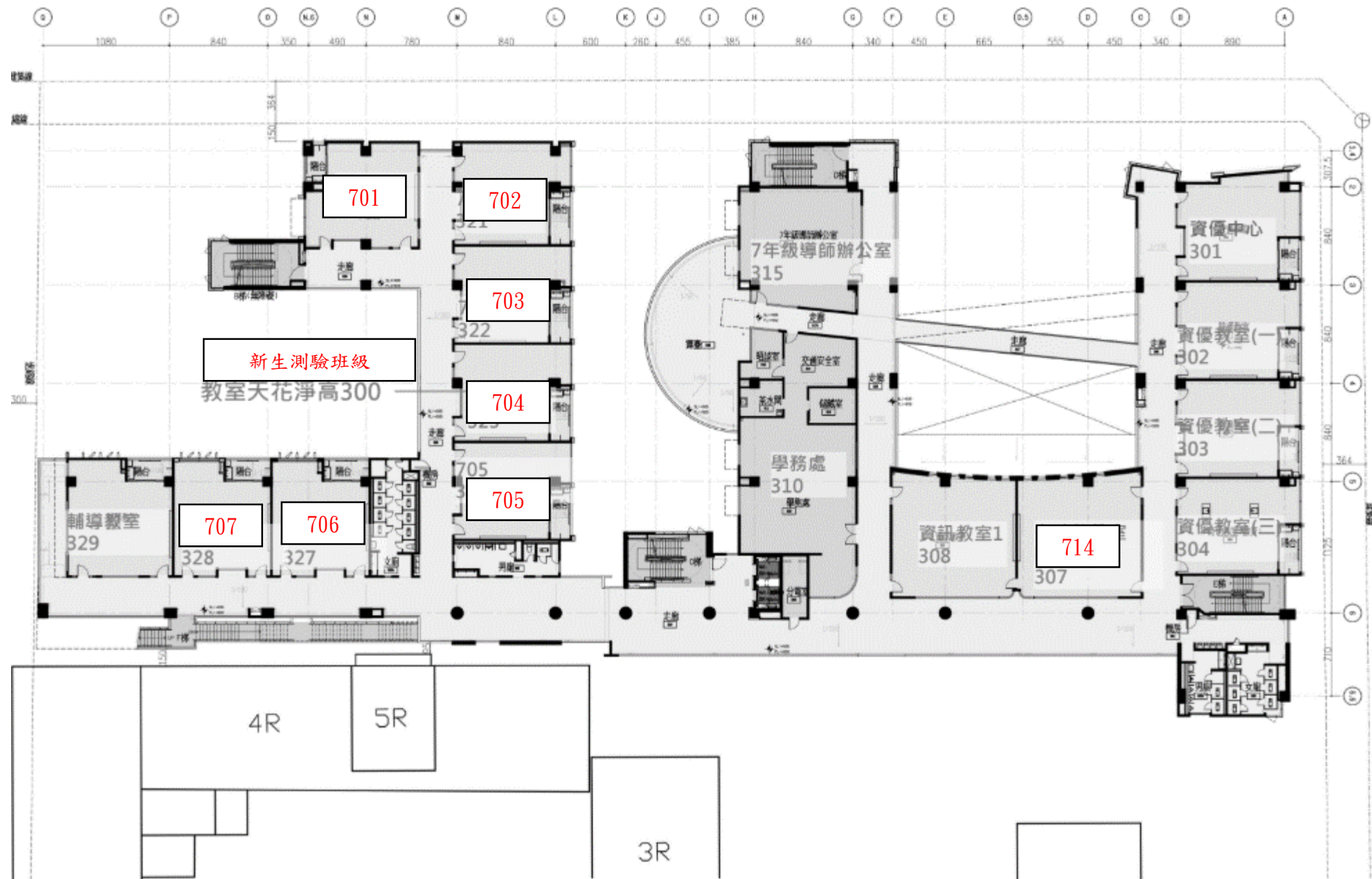
三層平面圖
